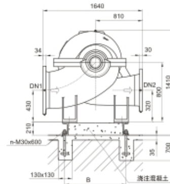
吸入法兰(Suction Flange)DN1及吐出管出口法兰 吐出法兰(Discharge Flange)DN2
