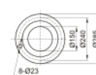
吸入法兰(Suction Flange)DN1 及吐出锥管出口法兰 吐出法兰(Discharge Flange)DN2
