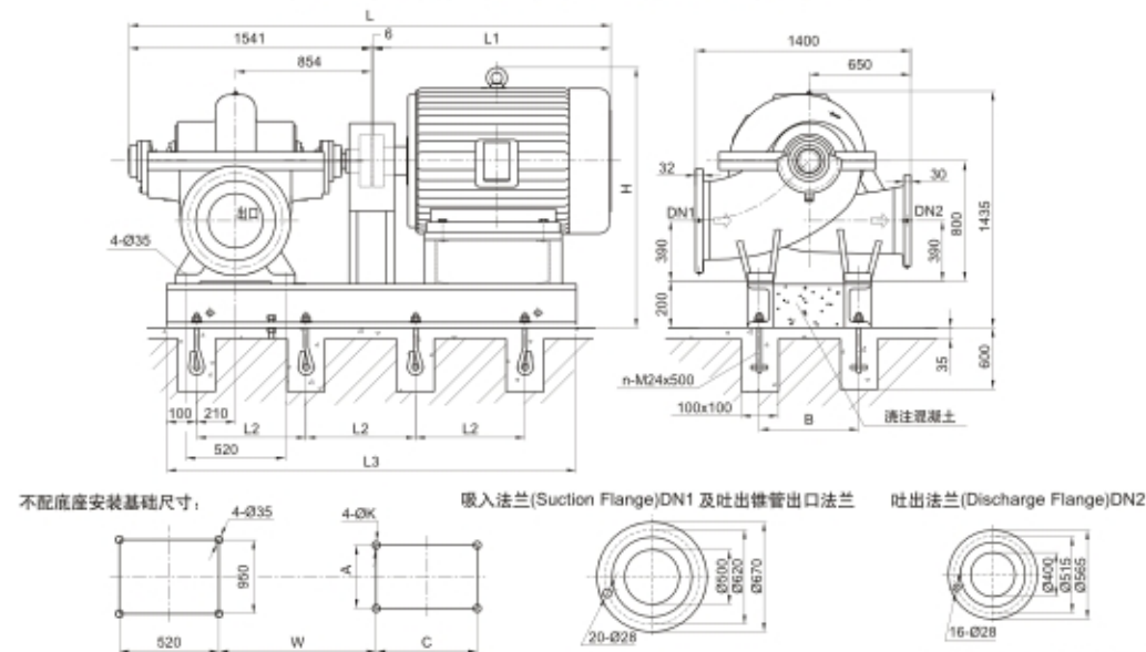
吐出接管长 E=300
