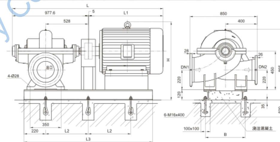
吸入法兰(Suction Flange)DN1 及吐出锥管出口法兰 吐出法兰(Discharge Flange)DN2
