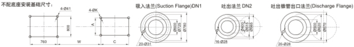
吐出锥管长 E=600
