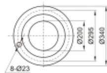
吸入法兰(Suction Flange)DN1 及吐出锥管出口法兰 吐出法兰(Discharge Flange)DN2
