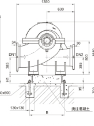
吸入法兰(Suction Flange)DN1及吐出管出口法兰
