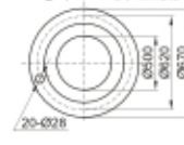
吸入法兰(Suction Flange)DN1及吐出管出口法兰 吐出法兰(Discharge Flange)DN2
