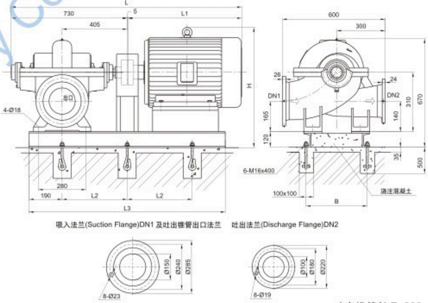
吐出锥管长 E=300
