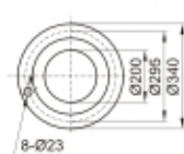
吸入法兰(Suction Flange)DN1 及吐出锥管出口法兰 吐出法兰(Discharge Flange)DN2
