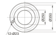
吸入法兰(Suction Flange)DN1 及吐出锥管出口法兰 吐出法兰(Discharge Flange)DN2
