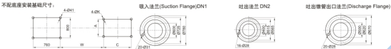
吐出锥管长 E=600
