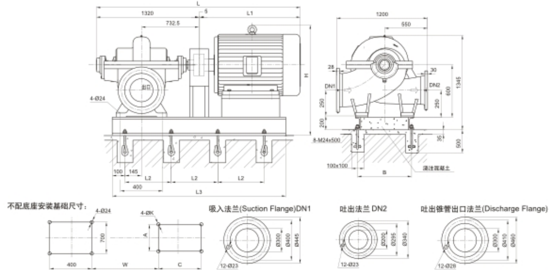
吐出锥管长 E=500
