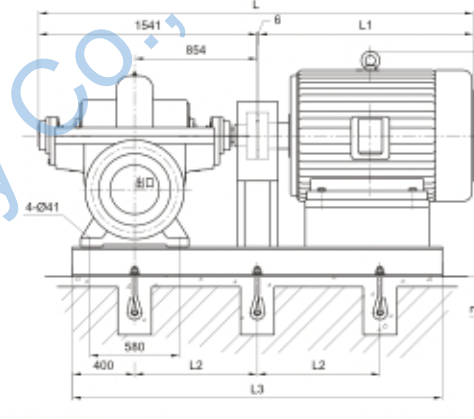
不配底座安装基础尺寸:
