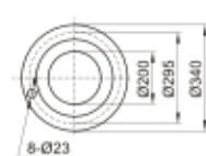
吸入法兰(Suction Flange)DN1 及吐出锥管出口法兰 吐出法兰(Discharge Flange)DN2
