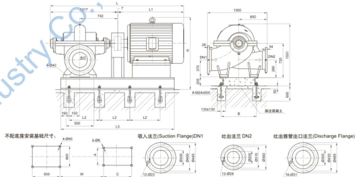
吐出锥管长 E=500
