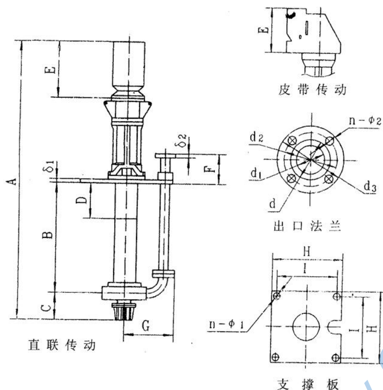
ZJL型渣浆泵安装图和安装尺寸表
