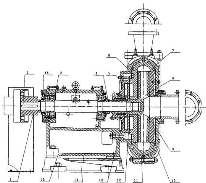
ZJ型渣浆泵结构图
