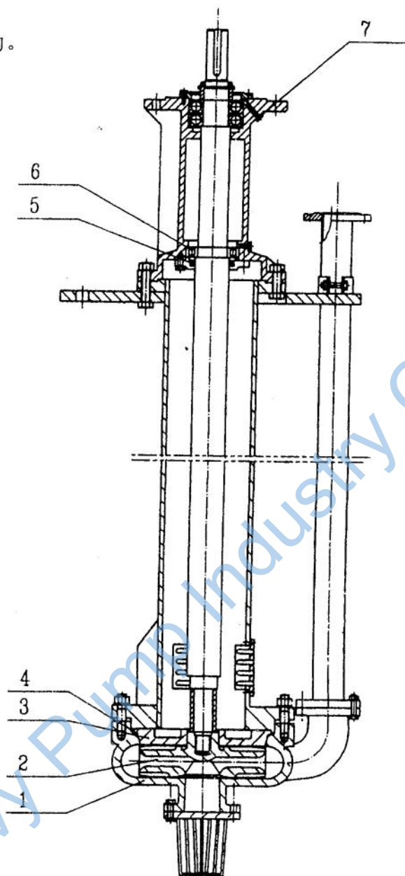
ZJL型渣浆泵结构图
