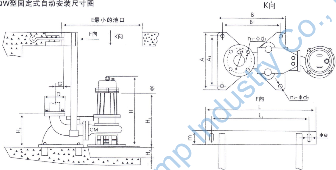
JYQW型固定式自动安装尺寸图
