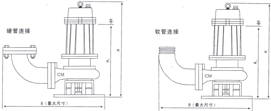
JYQW型移动式安装尺寸图
