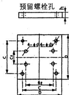
联接板
