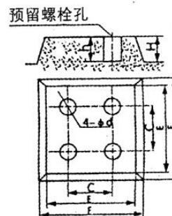
硬性联接基础图
