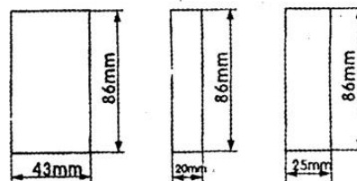
SD 型隔振垫 0.5 基本块尺寸
